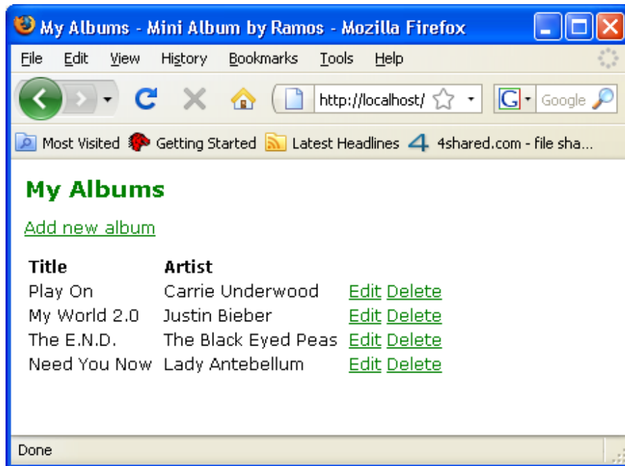
Gambar 1 Mini Album
